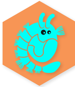
PUPA
